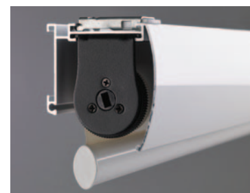
Molettes d'extrémités pour régler la tension du ressort et la position de la fin de course haute
