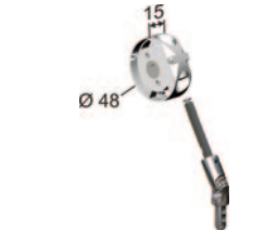
Détail des encombrements
