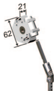
Treuil en zamak avec fin de course, rapport 5 : 1
