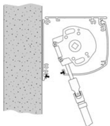
Sortie verticale sous coffre
