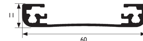
Section du profil support
