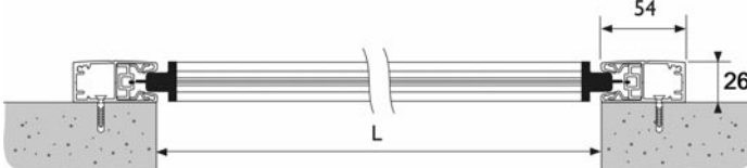
Coulisse zip tubulaire pour pose de face
