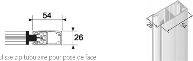
Coulisse zip tubulaire pour pose de face
