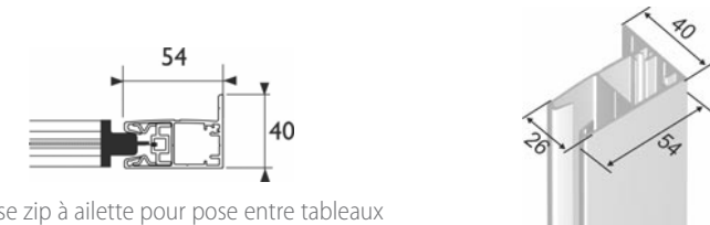
Coulisse zip à ailette pour pose entre tableaux
