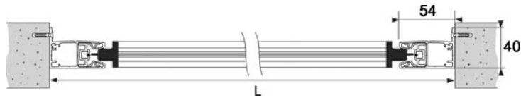
Coulisse zip à ailette pour pose entre tableaux
