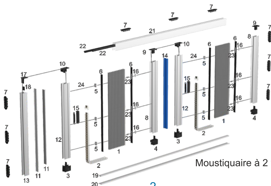
Moustiquaire à 2 vantaux opposés
